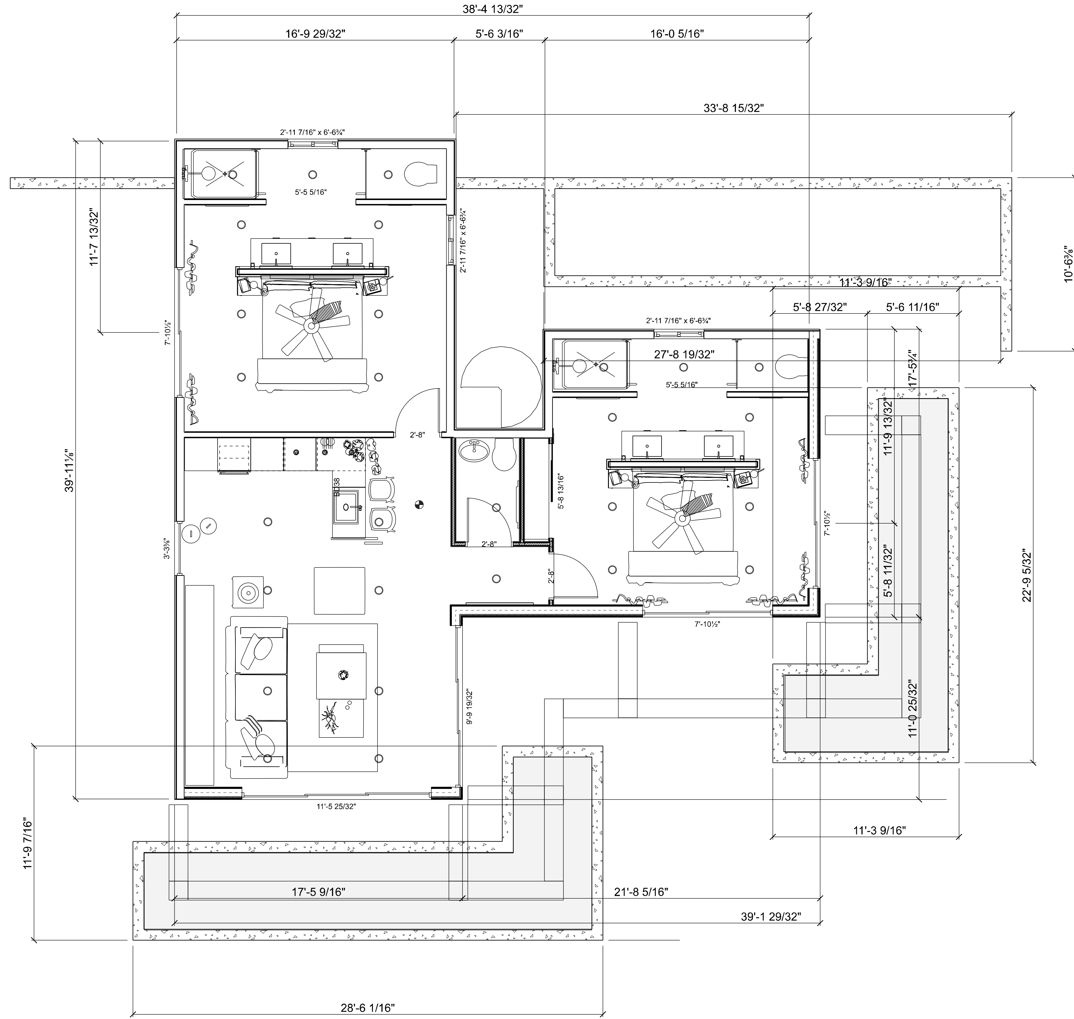
Tortola Luxe Floorplan SCALE: 0.2969" = 1'-0"
